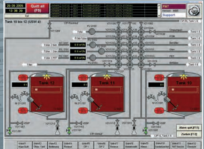
► Visualisierung Tanklager
